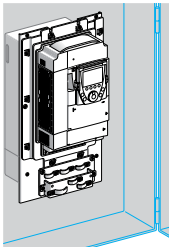
VW3 A95 Soğutucu ayırma montaj kiti
