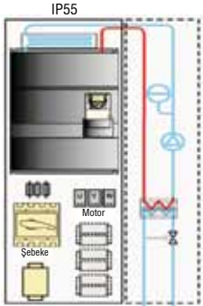
Su soğutmalı, panolu sürücü çözümü
