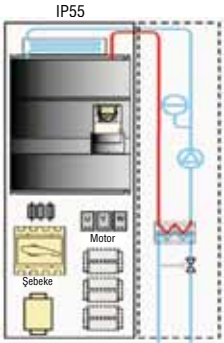
Su soğutmalı, panolu sürücü çözümü
