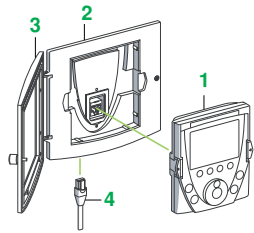
ATV61/71 uzaktan bağlantı kiti
